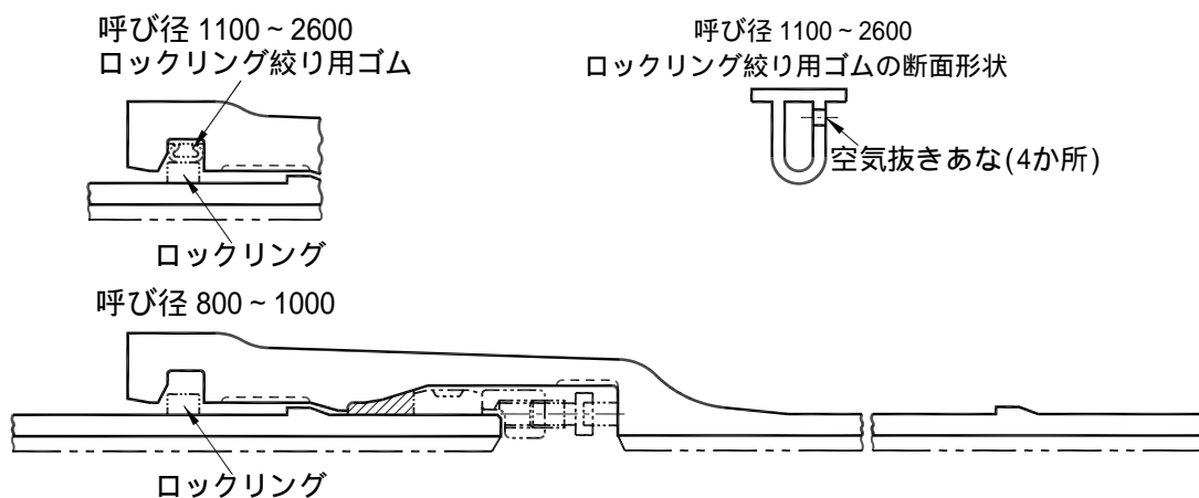
付表1 U S形ダクタイトイル鑄鉄管(L S方式)
