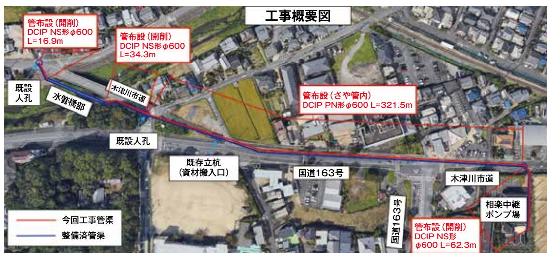
図1 工事概要
