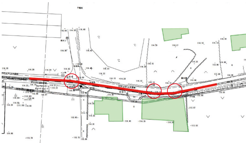
図4 平面図
