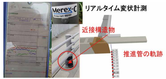
図7 距離確認と変位計測
