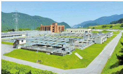
写真1 鶴来浄水場
