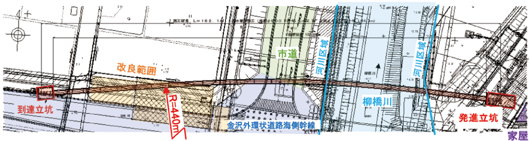
図2 平面図
