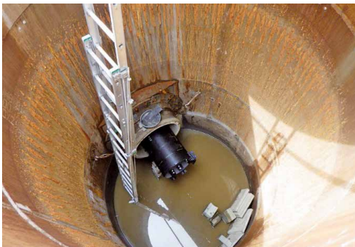
写真5 PN管到達状況
