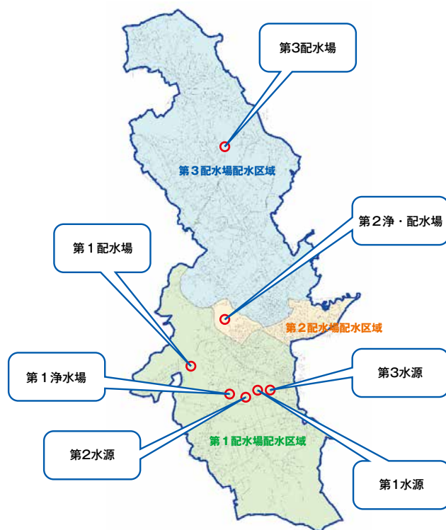
図2 給水区域図
