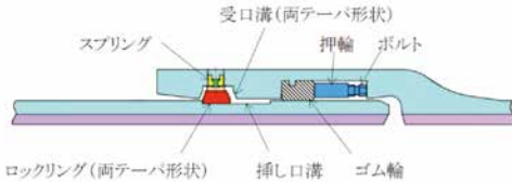
図7 PN形ダクタイトイル鉄管の継手構造
