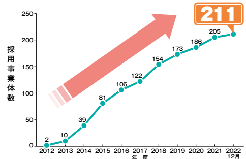
S50形ダクトイル鉄管の累計出荷実績と採用事業体数の推移
