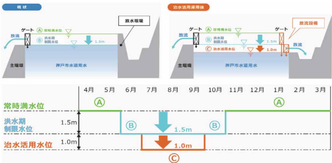
図4 千苜ダム 治水活用概要図
