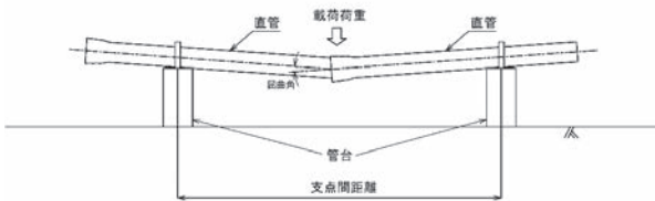
図8 曲げ試験方法
