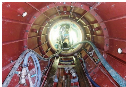
写真8 鋼製セグメント(曲線部)
