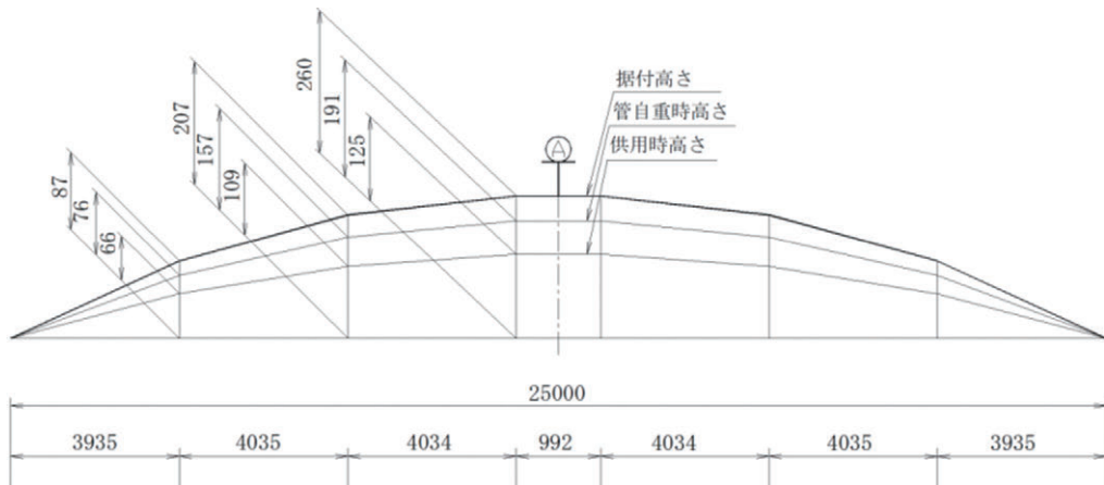
図5 水管橋キャンバ図
