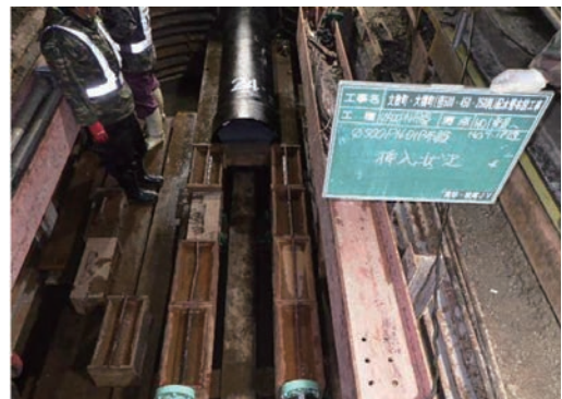
写真8 管挿入状況
