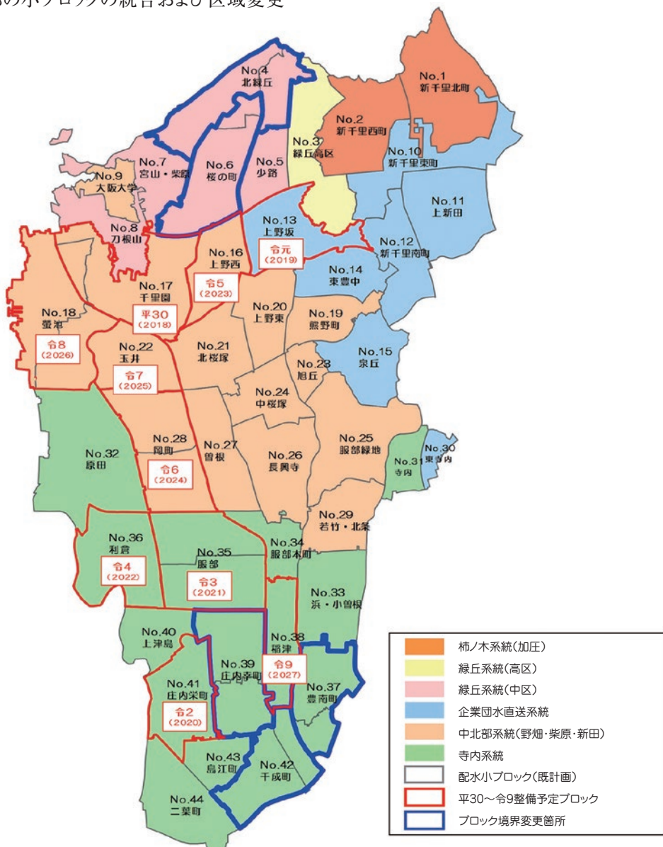
図12 配水小ブロックの整備計画図
