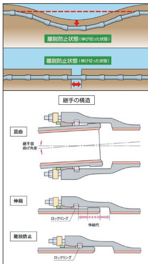
圖15 (2)案:鎖構造継手管路
