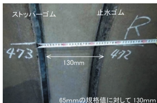
図5 継手部の抜け出し
