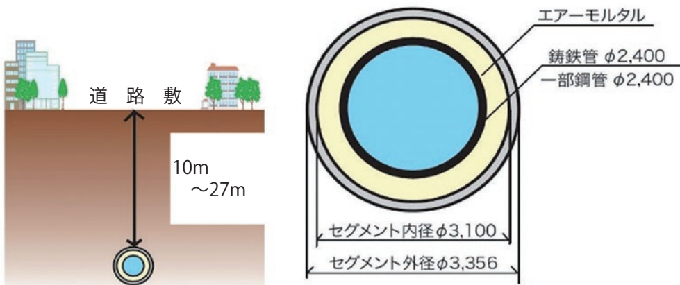
図4 標準断面図
