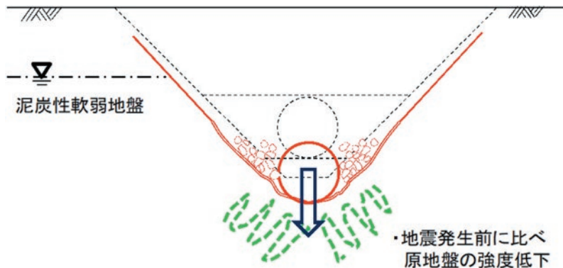
図13 軟弱地盤における管の不同沈下
