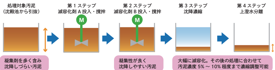
汚泥減容化フロー
