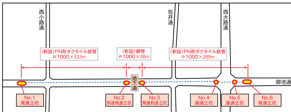
図7 その3工区の施工概要図
