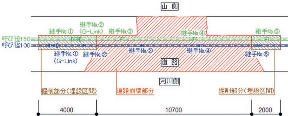
図3 工事範囲
