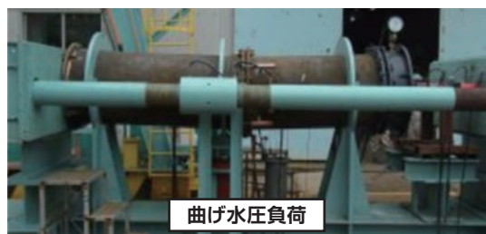
写真4 水密性試験状況
