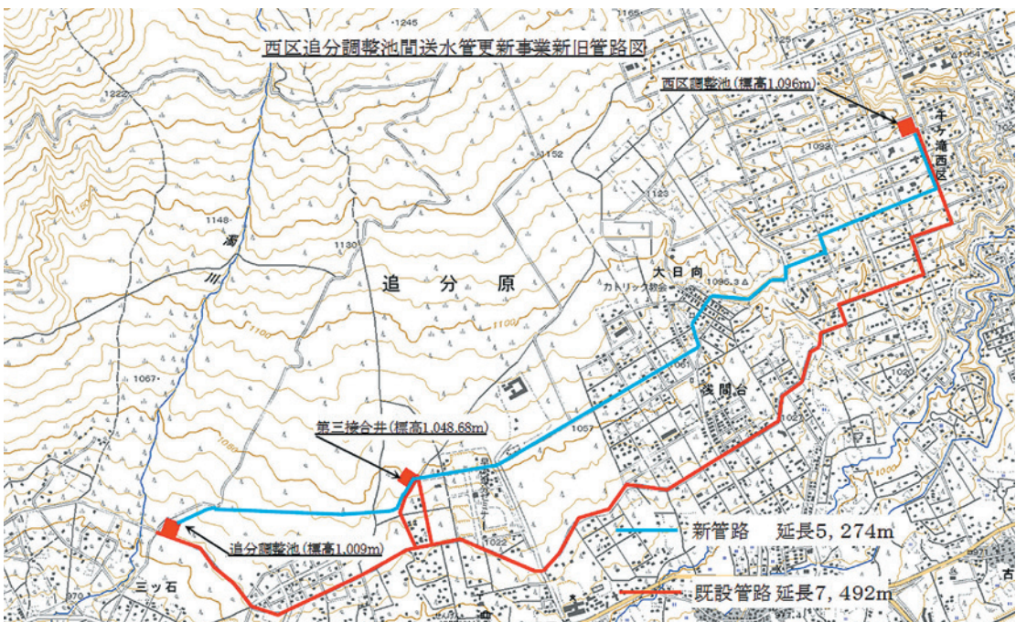
図3 新旧管路図
