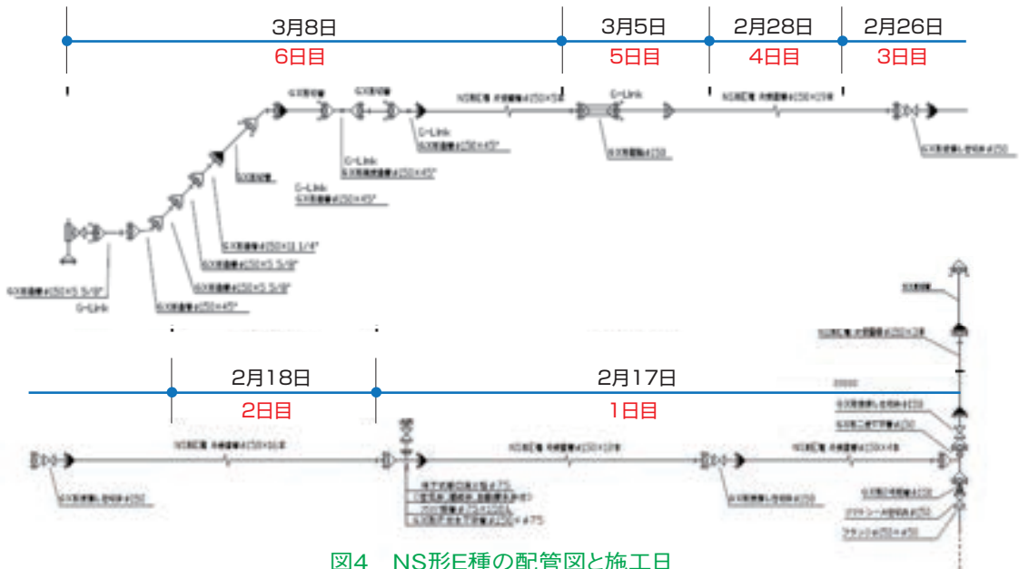
図4 NS形E種の配管図と施工日
