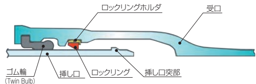
図2 プッシュオンタイプ(GX形直管)
