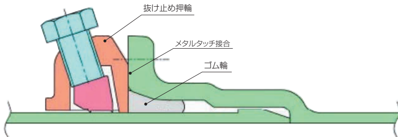
図5 離脱防止構造(S50形)
