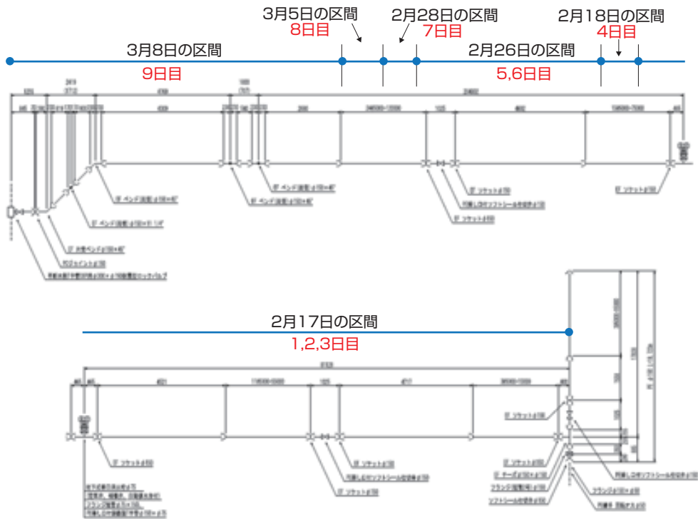
図5 水道配水ポリエチレン管の計画配管図と作業推定日数
