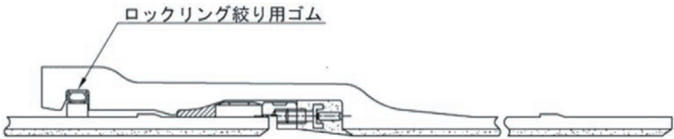
図5 US形継手構造図(LS方式)
