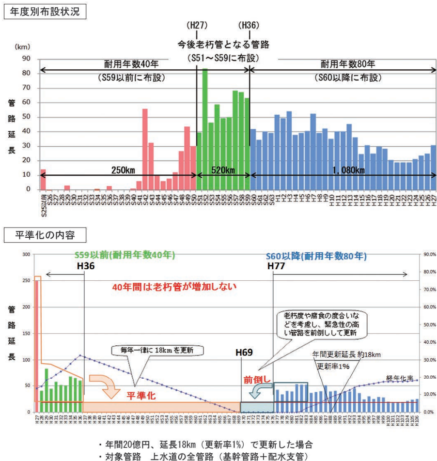
図8 老朽管更新事業計画
