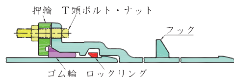
図 1 直管の構造
