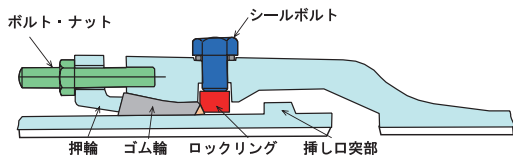
図 4 開発当初の耐震継手構造の一例
