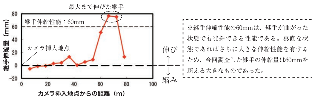
図 24 継手伸縮量の調査結果
