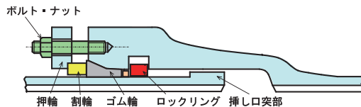
図 6 S 形継手 (現在) の構造
