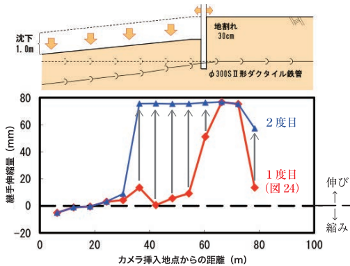
図 26 2度目の地震に対するシミュレーション結果 (呼び径300 SⅡ形管路)
