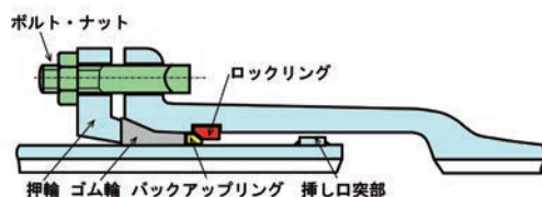
図 12 S II 形継手
