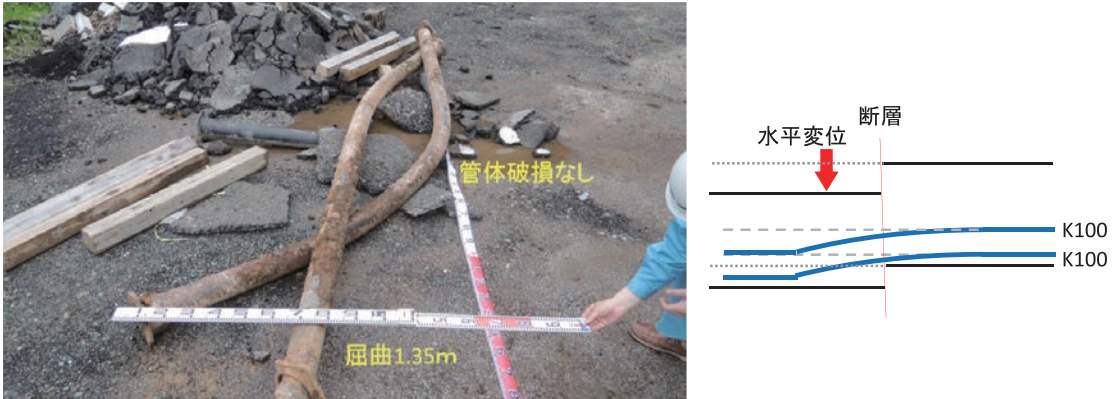
図7 断層横断部の管路被害状況(益城町下陳) ＜呼び径100K形ダクタイル鉄管＞
