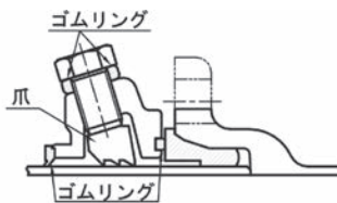
図8 异形管受口に切管を接合する場合 (N-Link を使用)
