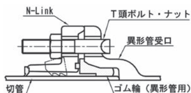
図8 异形管受口に切管を接合する場合 (N-Link を使用)
