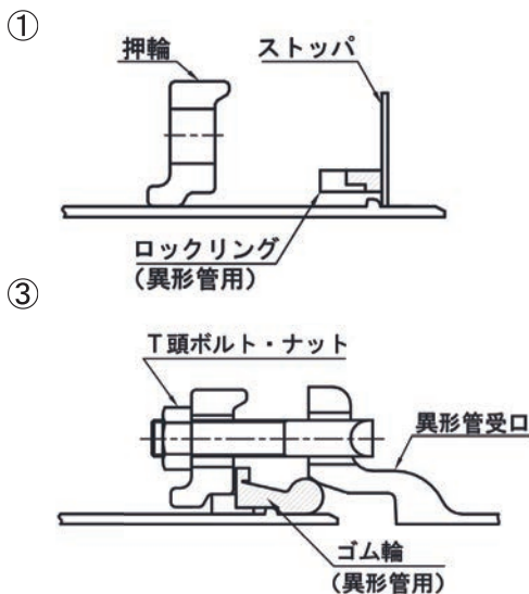
図9 異形管の接合手順
