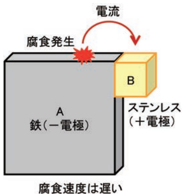
図8-3 腐食速度のイメージ図
