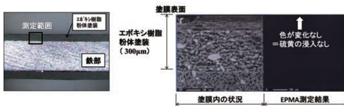
図Ⅱ-1 硫黄侵入深さの結果(エポキシ樹脂粉体塗装)
