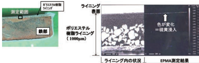
図Ⅱ-2 硫黄侵入深さの結果(参考:ポリエステル樹脂ライニング)
