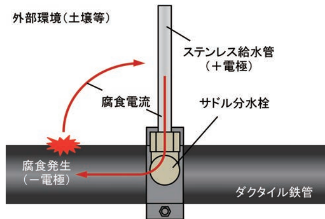
図9 ステンレス給水管とダクトイル鉄管の異種金属腐食の一例
