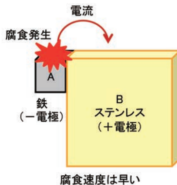
図8-3 腐食速度のイメージ図
