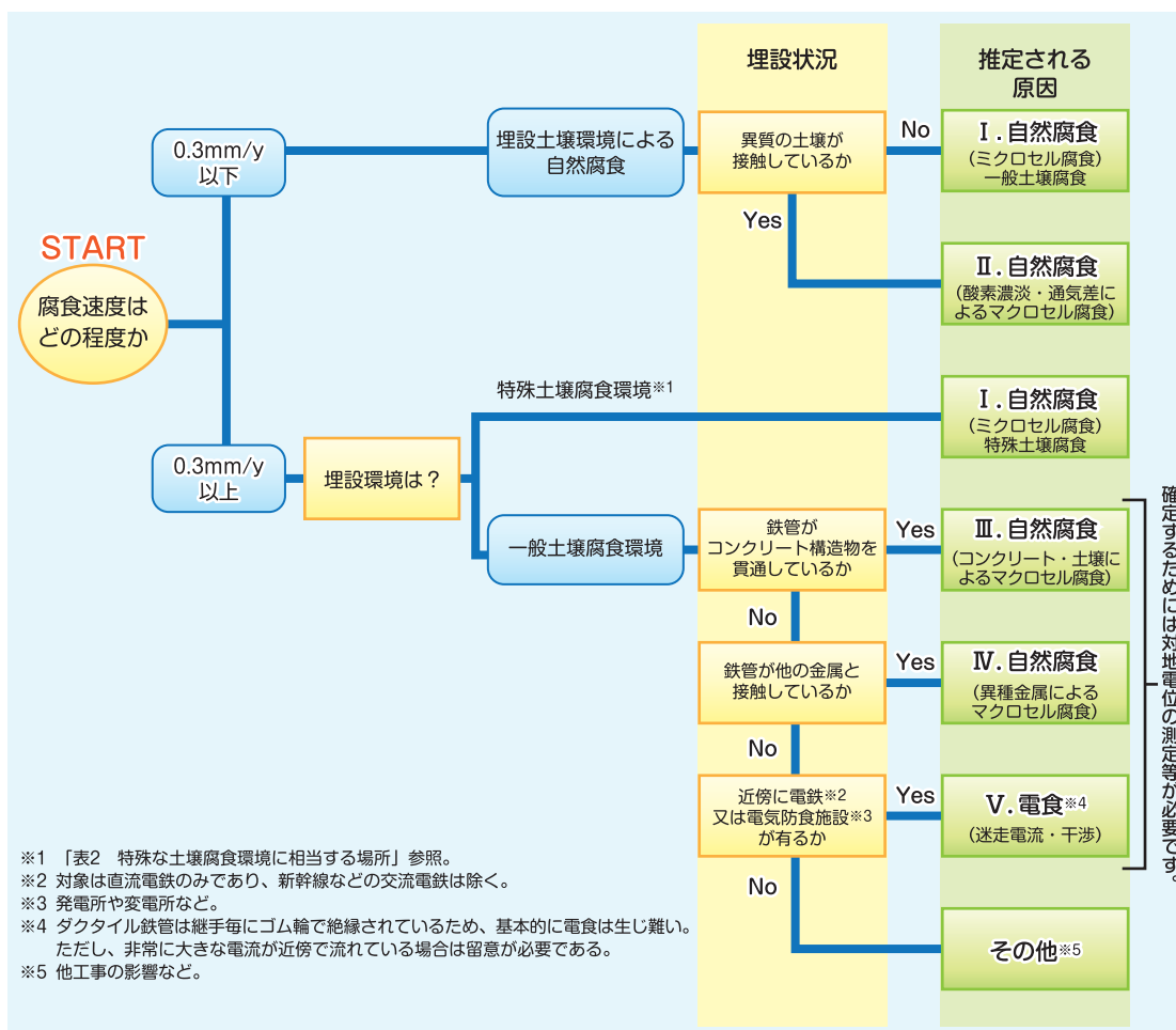
図3 腐食原因推定フローチャート
