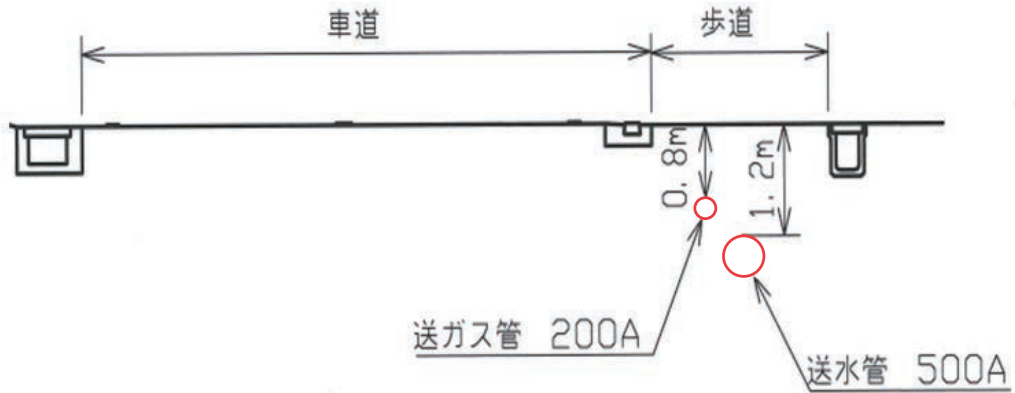
図7 一般断面図
