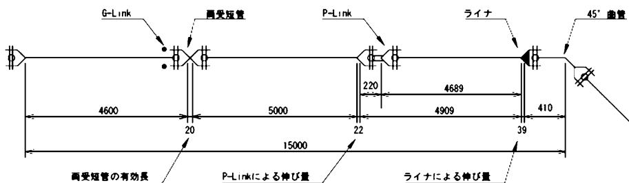
図3 寸法記入例
