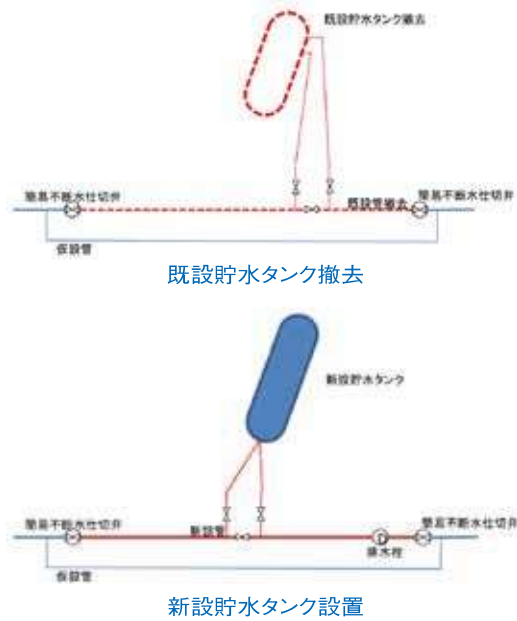
図7 施工手順
