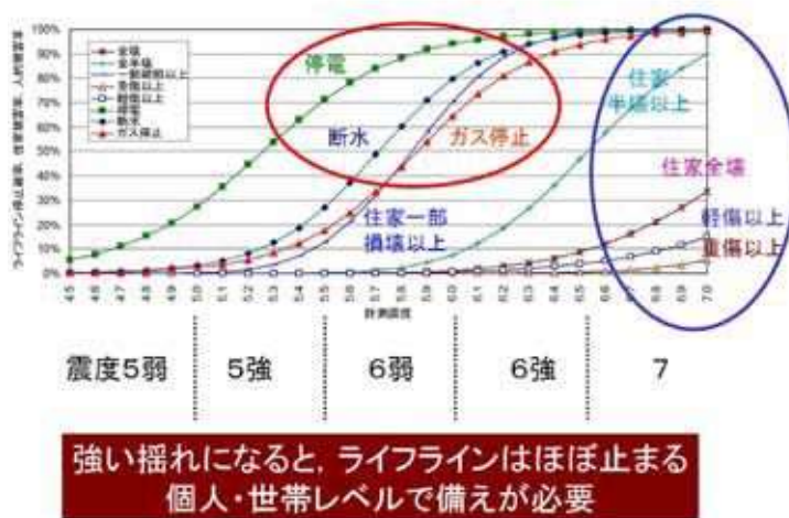
図7 震度と被害のおおよその関係
