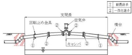
図2 ダクタイトル水管橋(長支間の場合、タイプⅡ)
