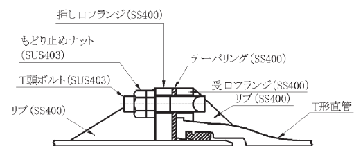
図6 FT形継手 (呼び径75~350)
