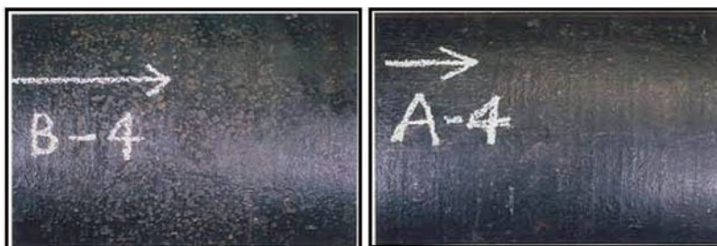
写真No1 埋設20年後の管外面の状況
