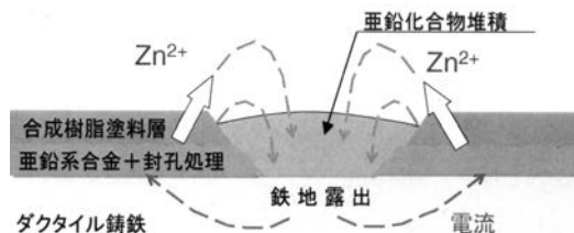
図5 自己防食のメカニズム
