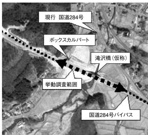
図2 国道284号バイパス
