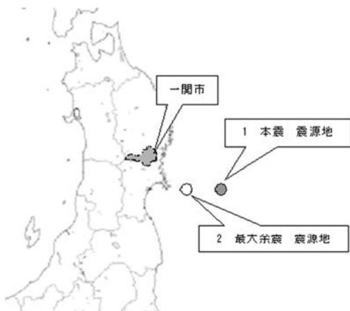
図1 一関市と震源の位置関係および震度概要
