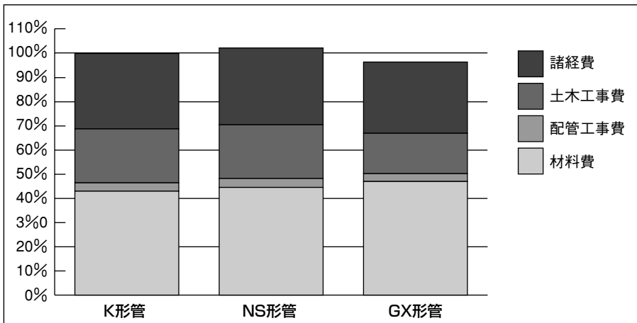
図2 呼び径250配管工事比較
