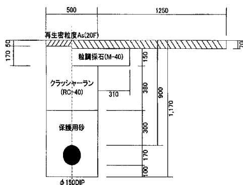
図7 掘削断面
