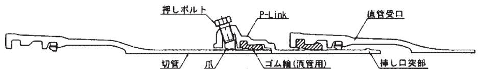
図1 P-Linkを使用したGX形直管の継手構造
