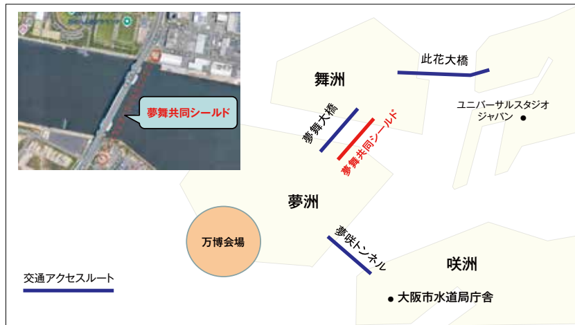
図2 夢舞共同シールド(海底トンネル)の位置図
