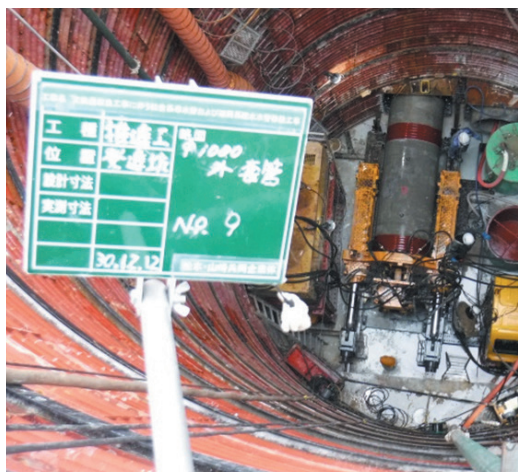
写真2 φ1000ヒューム管推進状況
