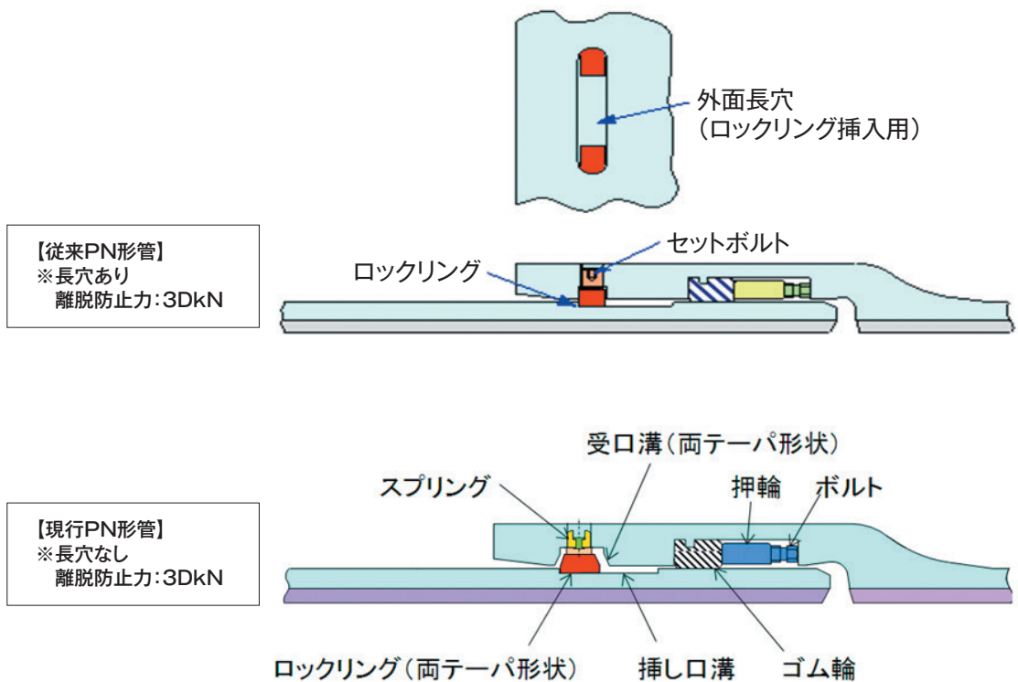
図5 PN形ダクトイル鉄管の継手構造
