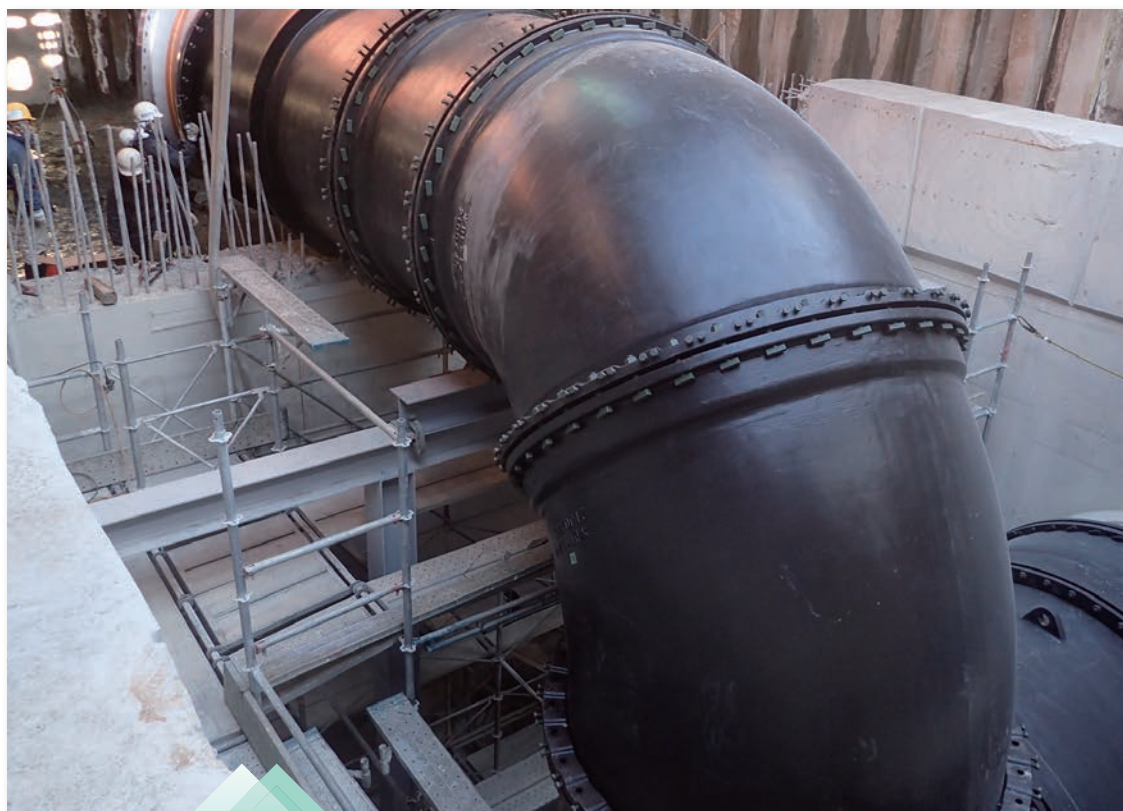
埼玉県荒川左岸南部下水道事務所 K形曲管 呼び径2100
