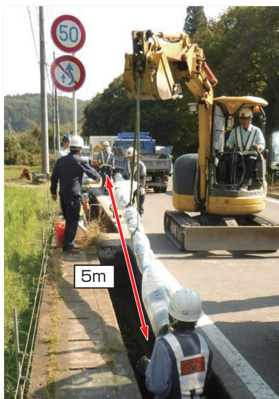
栃木県 芳賀中部上水道企業団 NS形E種 呼び径 100 (5m)
