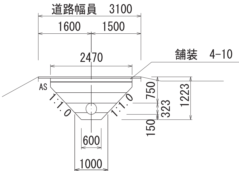
図3 施工断面(例)
