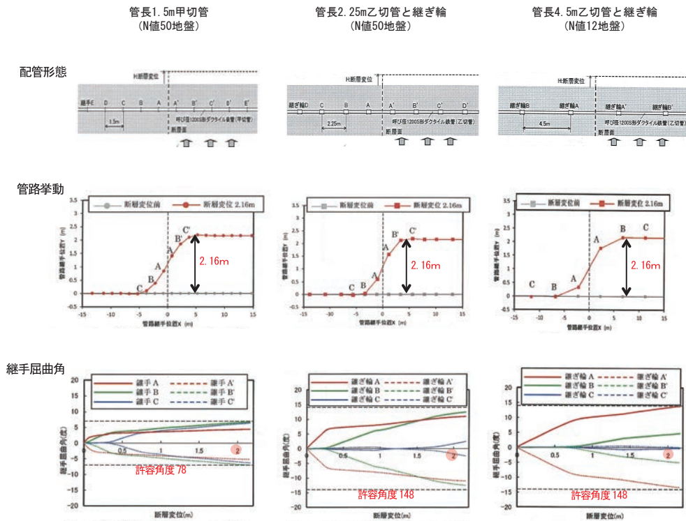
図8 2.16mの断層変位による管路挙動と継手屈曲の検証
