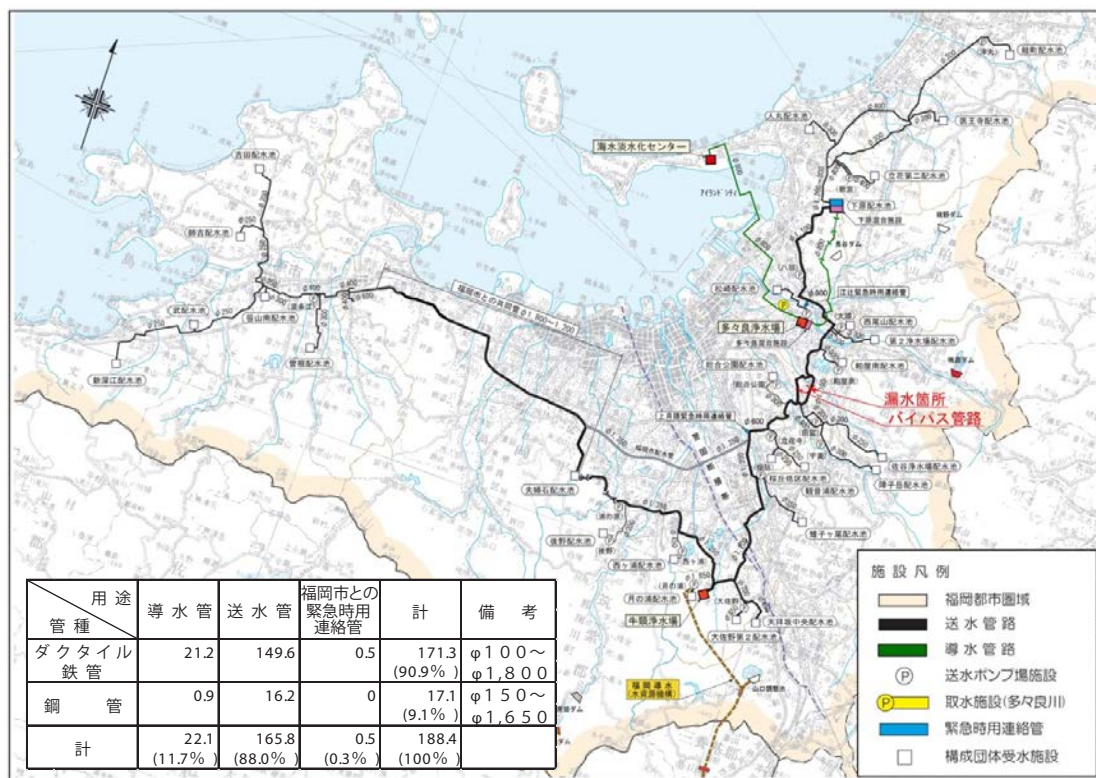
図2 施設整備概要図
