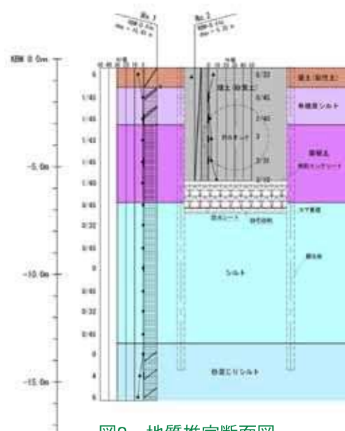
図2 地質推定断面図
