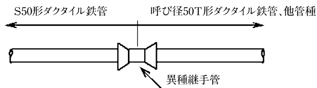
図1 呼び径50T形ダクタイトイル鉄管や他管種との接続方法例
