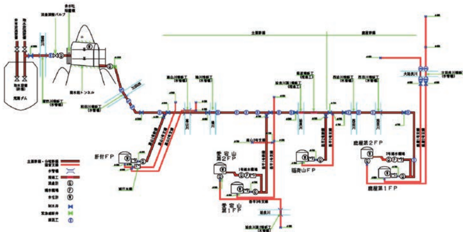
図2 農業用水の送配水体系
