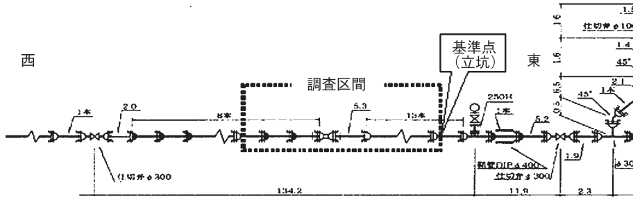
図3 調査対象管路①の概要
