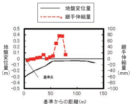
図12 管路挙動と地盤変位の比較
