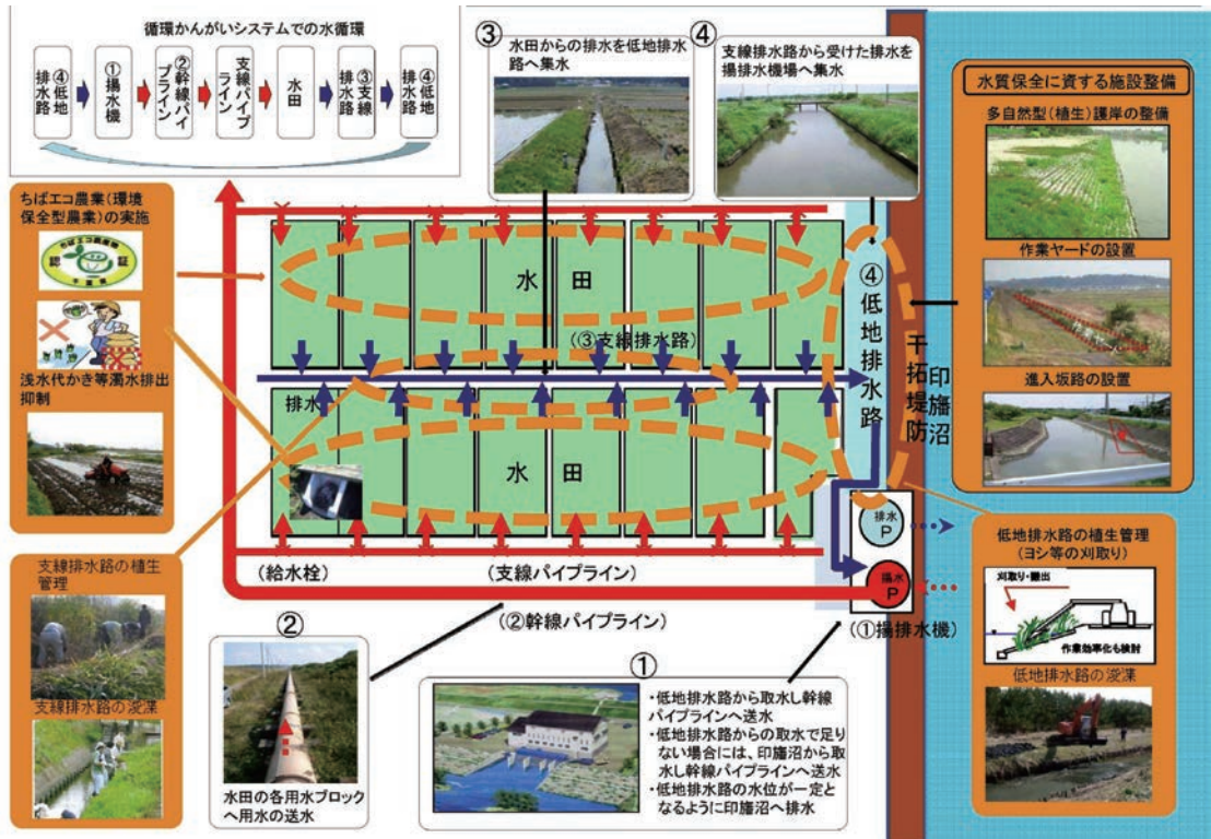
図2 循環かんがいシステムのイメージ
