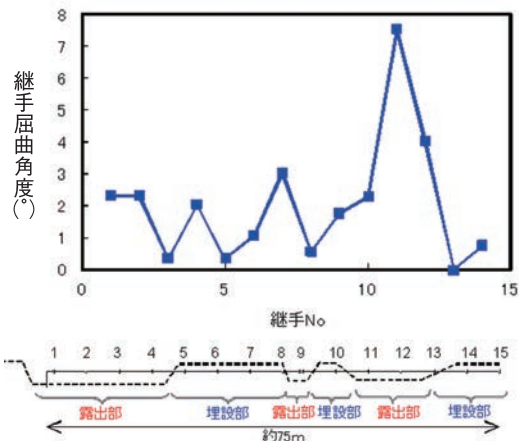
図14 各継手の屈曲角の測定結果
