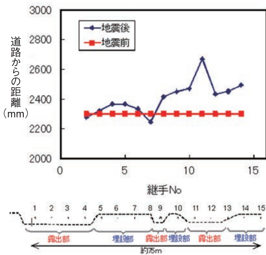
図13 道路端と管路の距離の測定結果
