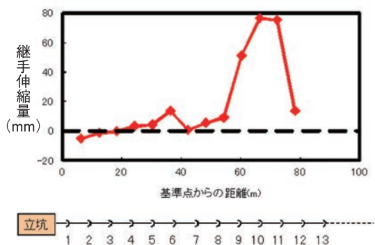
図11 継手伸縮量の算出結果
