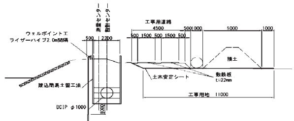
図3 標準断面図
