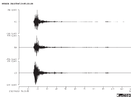
図2 時刻歴加速度波形、応答スペクトル（K-NET五色） (引用:独立行政法人 防災科学技術研究所ホームページ)
