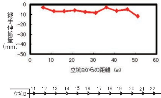
図16 継手伸縮量の測定結果(管路B)
