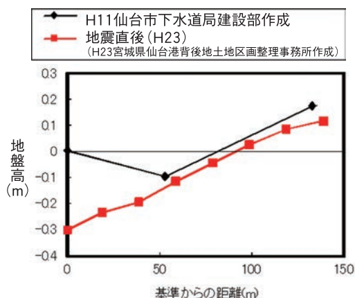
図10 地盤高の測量結果
