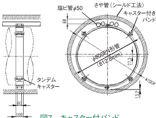
図7 キャスター付バンド
