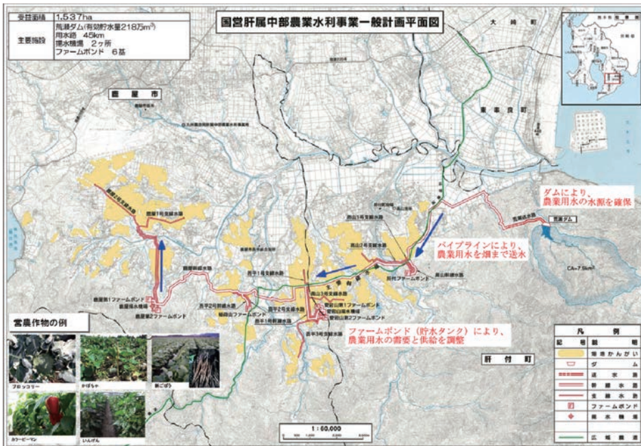
図1 国営肝属中部農業水利事業の一般計画平面図
