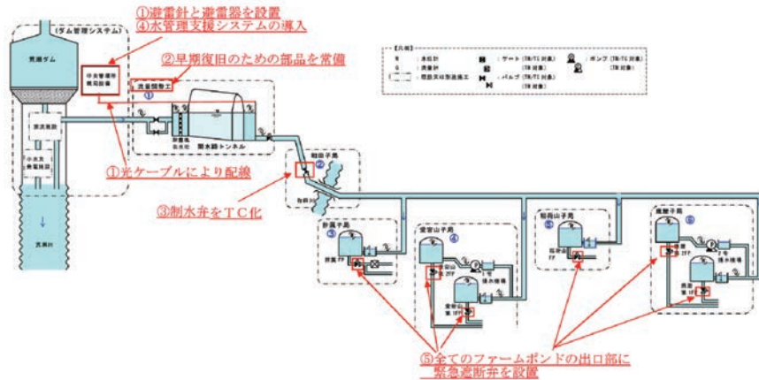
図5 リスクマネジメントの検討を取り入れた農業水利施設の設計
