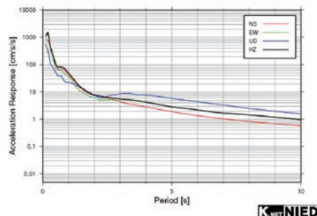
図2 時刻歴加速度波形、応答スペクトル（K-NET五色） (引用:独立行政法人 防災科学技術研究所ホームページ)
