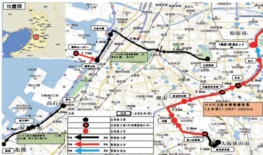
図3 バイパス送水管位置図
