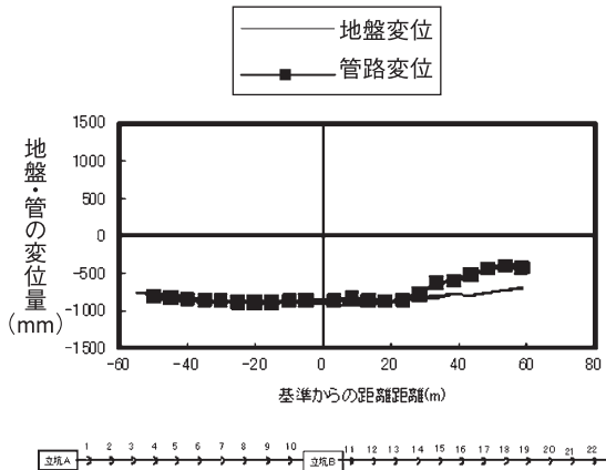
図17 地震後の地盤と管路の変位量
