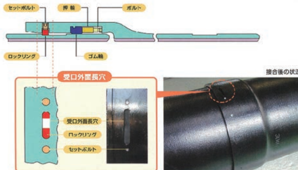
図3 PN形管の継手構造
