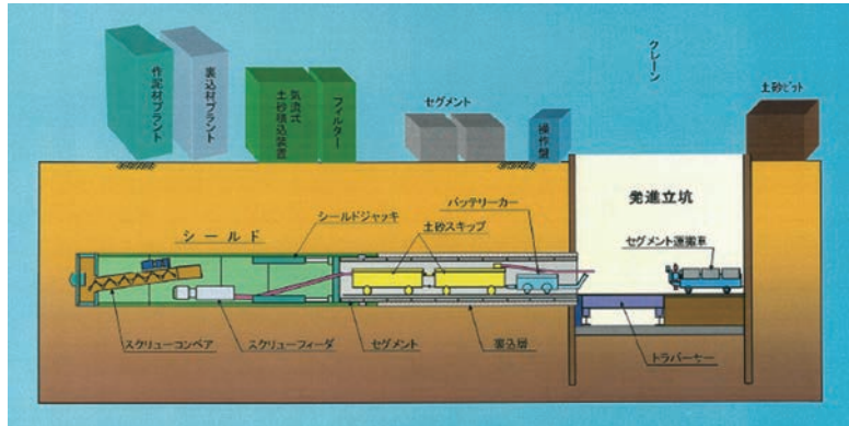
図9 シールド工法概念図
