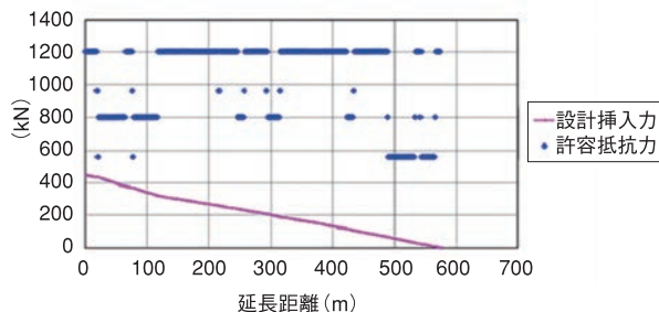
図8 設計挿入力と許容抵抗力 (標準タイプ)
