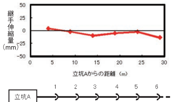
図15 継手伸縮量の測定結果(管路A)
