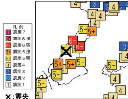
図1 淡路島付近の地震における各地の震度 〈淡路島付近の拡大図〉 (引用:気象庁ホームページ)
