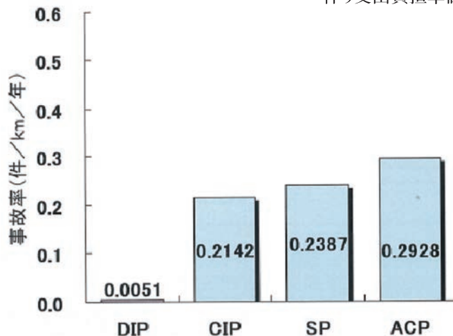
図4 管種別のパイプラインの事故率
