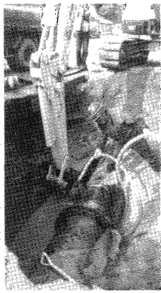
昭和30年代の700m口径鉄管の復旧を急ぐ(いわき市)
