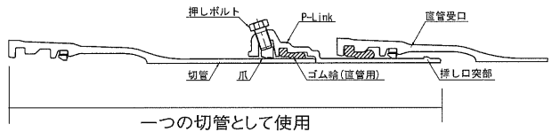
図4 P-Linkの構造
