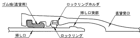
図2 GX形直管の継手構造
