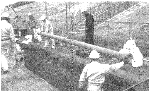
写真1 呼び径150GX形の吊り込み状況
