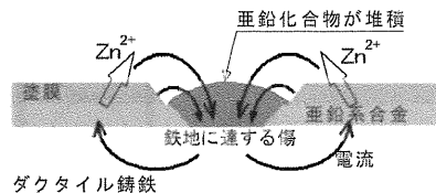
図6 傷部の防食のメカニズム
