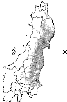
図1 震度マップ 1)
