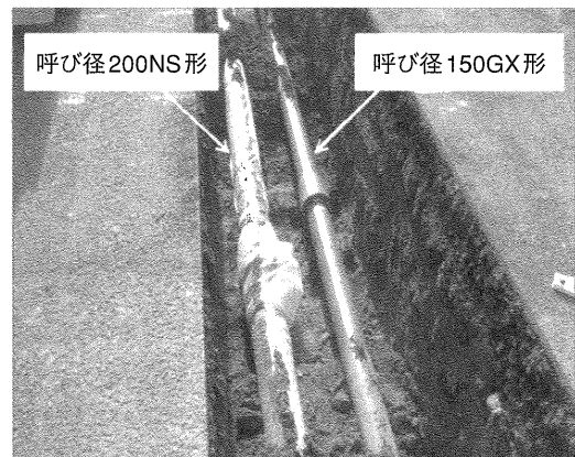
写真3 呼び径150GX形の据付完了 (配水管呼び径200NS形との2条配管)
