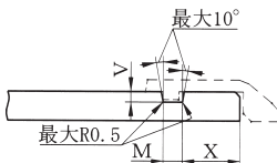
切管挿し口
