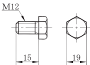
ライナ用ボルト c)
