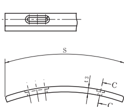
挿しロリング用結合ピース a) (SUS304)
