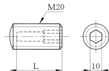
ライナ心出し用ボルト
