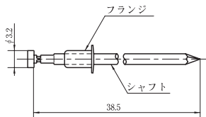
リベット b)
