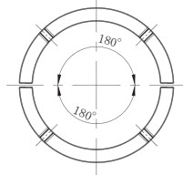
呼び径600・700 (3分割)
