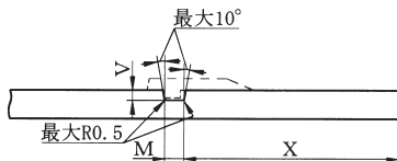
切管挿し口
