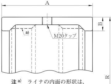
断面 A-A
