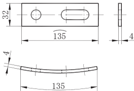
ライナ用留め具 b)
