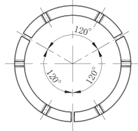
呼び径800～1000 (4分割)
