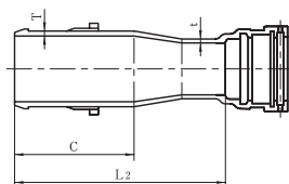
呼び径 100 ~ 250
