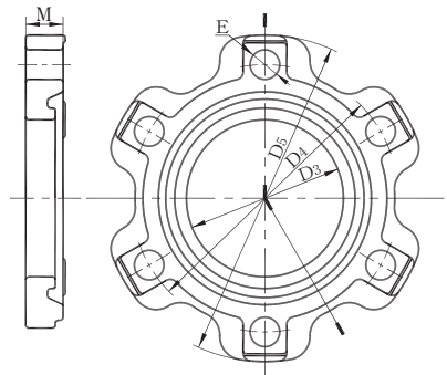
呼び径400・450
