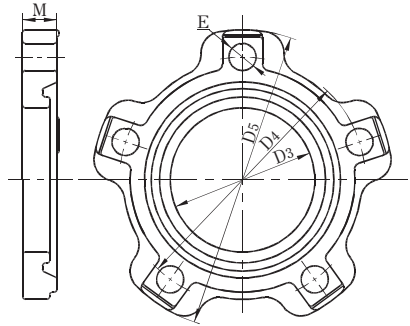
呼び径350
