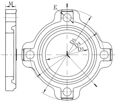
呼び径300
